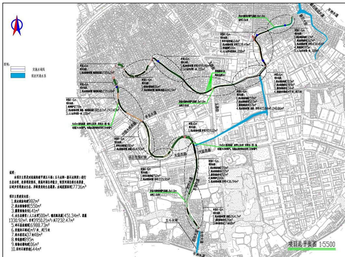
工艺平面布置图
